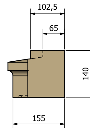
'PW' TYPE PROFILE ( 1 : 5 )
