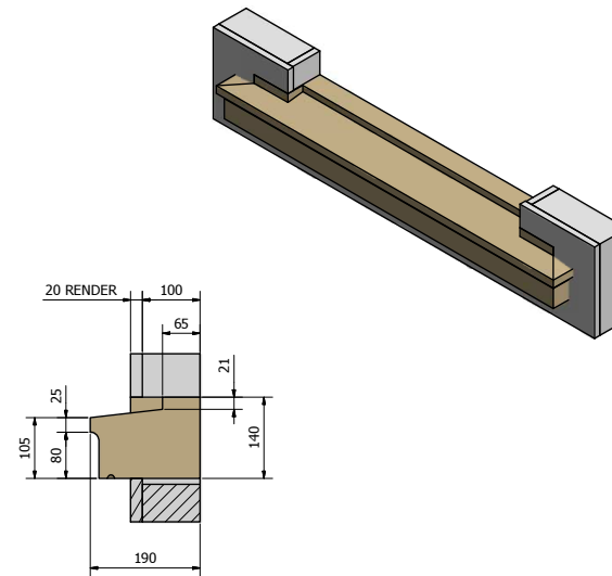
A-A ( 1:5 )
