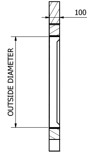
'RND' SECTION ( 1 : 15 )
