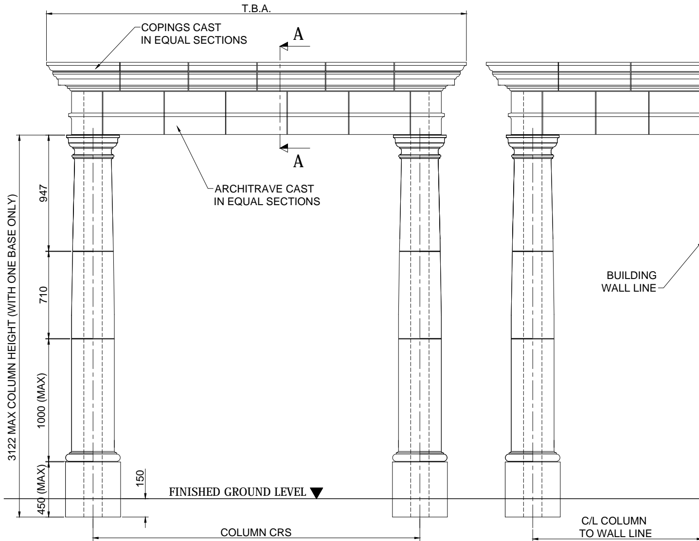
ELEVATION
